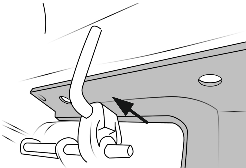
6.1 Установить глушитель install exhaust system
